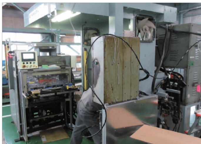
改造後磁気探傷装置
